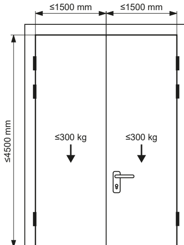
Abb. 3: Max. Türmaße und Gewichte
