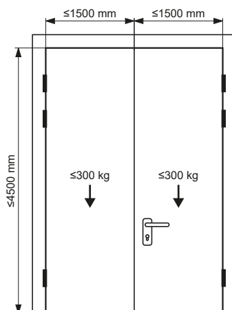
Fig. 3 : cotes et poids max. de la porte
