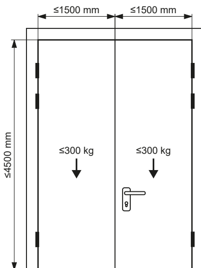
Fig. 3: dimensiones y pesos de puerta máx.
