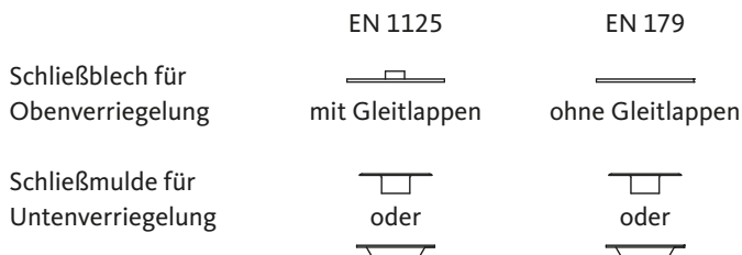
Abb. 2: Zulässige Schließblechkonturen
