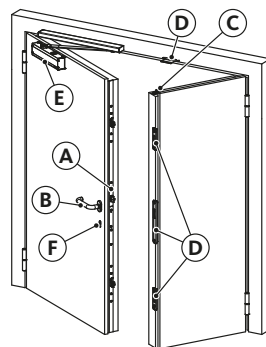
Fig.1: componentes del dispositivo
